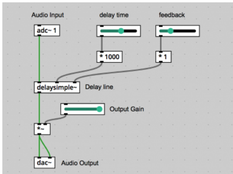
Figure 2. Patch Kiwi appliquant un retard avec réinjection et un gain sur un signal audio
